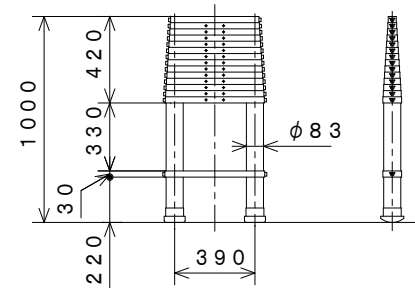
収納時寸法 (全15段)
